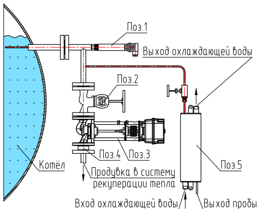
Рис.1 — Стандартная комплектация верхней продувки PRO-ES V1 (V2) .
