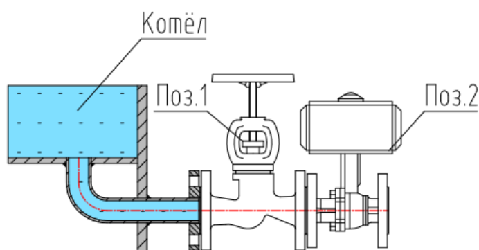
Рис.2 — Стандартная комплектация нижней продувки PRO-ES N .
